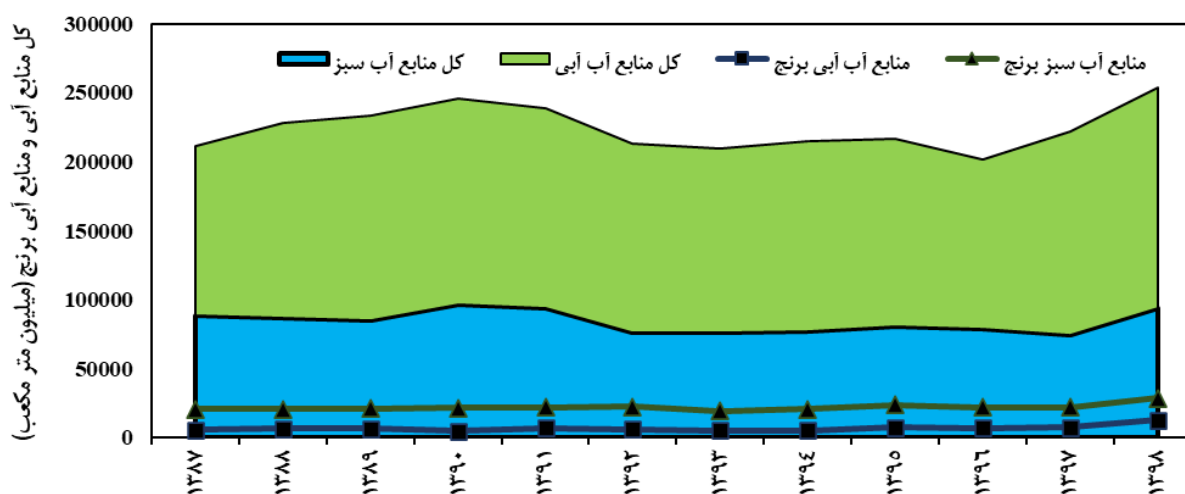
شکل ۴- منابع آب در دسترس کشاورزی و منابع آب در دسترس برای تولید برنج در ایران طی دوره آماری ۱۳۸۷ تا ۱۳۹۸
