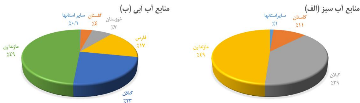
شکل ۳- منابع آب آبی و سبز در دسترس برای تولید برنج در ایران طی دوره آماری ۱۳۸۷ تا ۱۳۹۸
