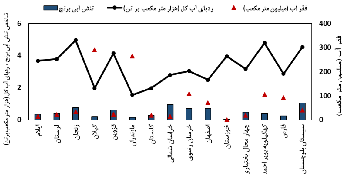
شکل ۱۰- تغییرات ردپای آب و شاخص‌های تنش آبی و فقر آب در تولید برنج در ایران Figure 10- Changes in the water footprint and indicators of water stress and water poverty of rice crop in Iran
