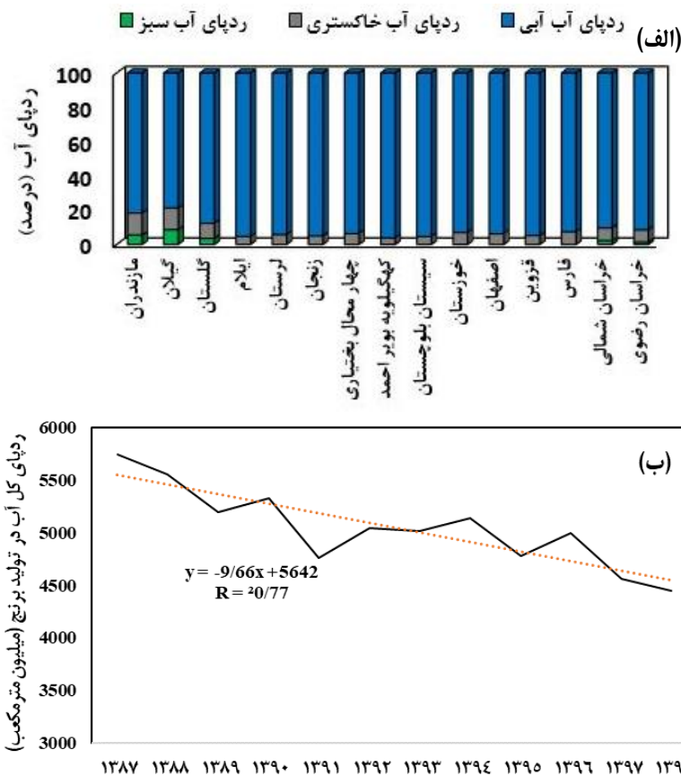
شکل ۶- سهم اجزاء ردپای آب (الف) و تغییرات زمانی ردپای آب در محصول برنج در مقیاس استانی و ملی (ب)
