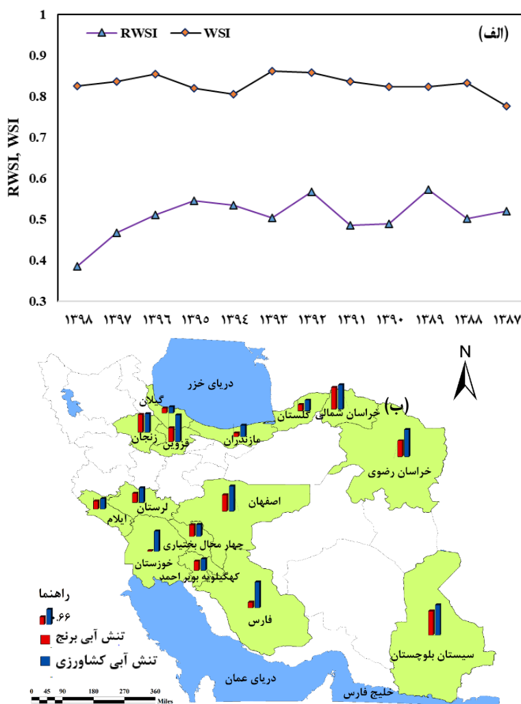
شکل ۸- تغییرات مکانی (الف) و زمانی (ب) شاخص تنش آبی کشاورزی و تنش آبی برنج در مقیاس استانی و ملی
