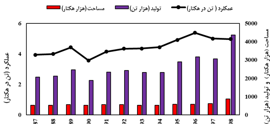
شکل ۲- متوسط سطح زیرکشت، تولید و عملکرد برنج در ایران طی دوره آماری ۱۳۸۷ تا ۱۳۹۸
