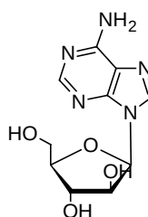
(16) Ara A
