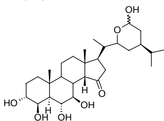
(15) Contignasterol
