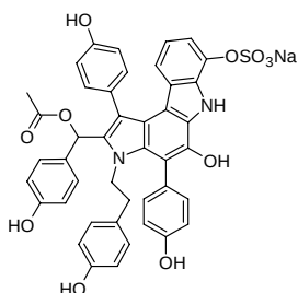
(4) Dictyodendrin A
