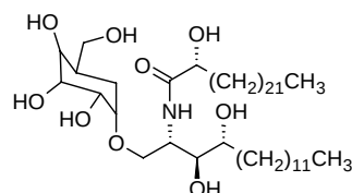
(9a) Agelasphin
