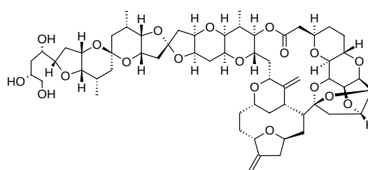
(7a) Halichondrin B
