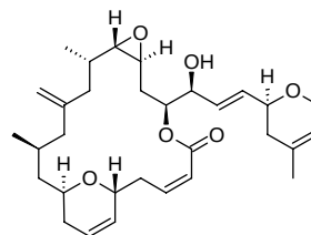
(3) Peloruside A
