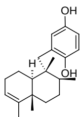
(13) Avarol
