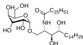
(9) KRN 7000
