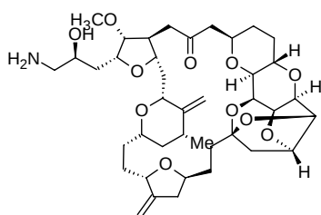
(7): E7389
