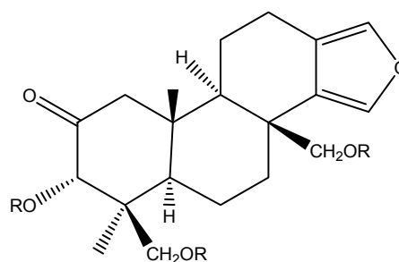
95. R=H 99. R=Ac
