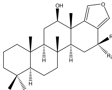
313. R_1=H , R_2=OH
